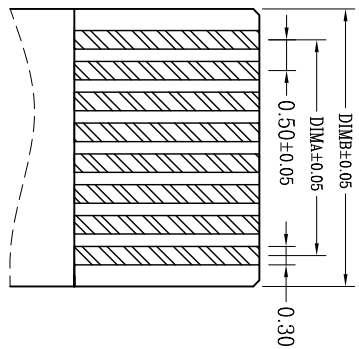
适用扁平线
