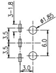
P.C.B LAYOUT
