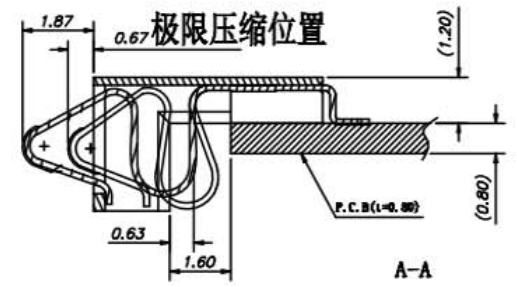
剖视图
