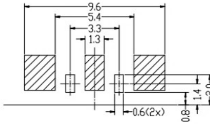
P.C.B LAYOUT
