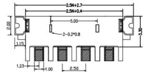
PCB LAYOUT(4pin)
