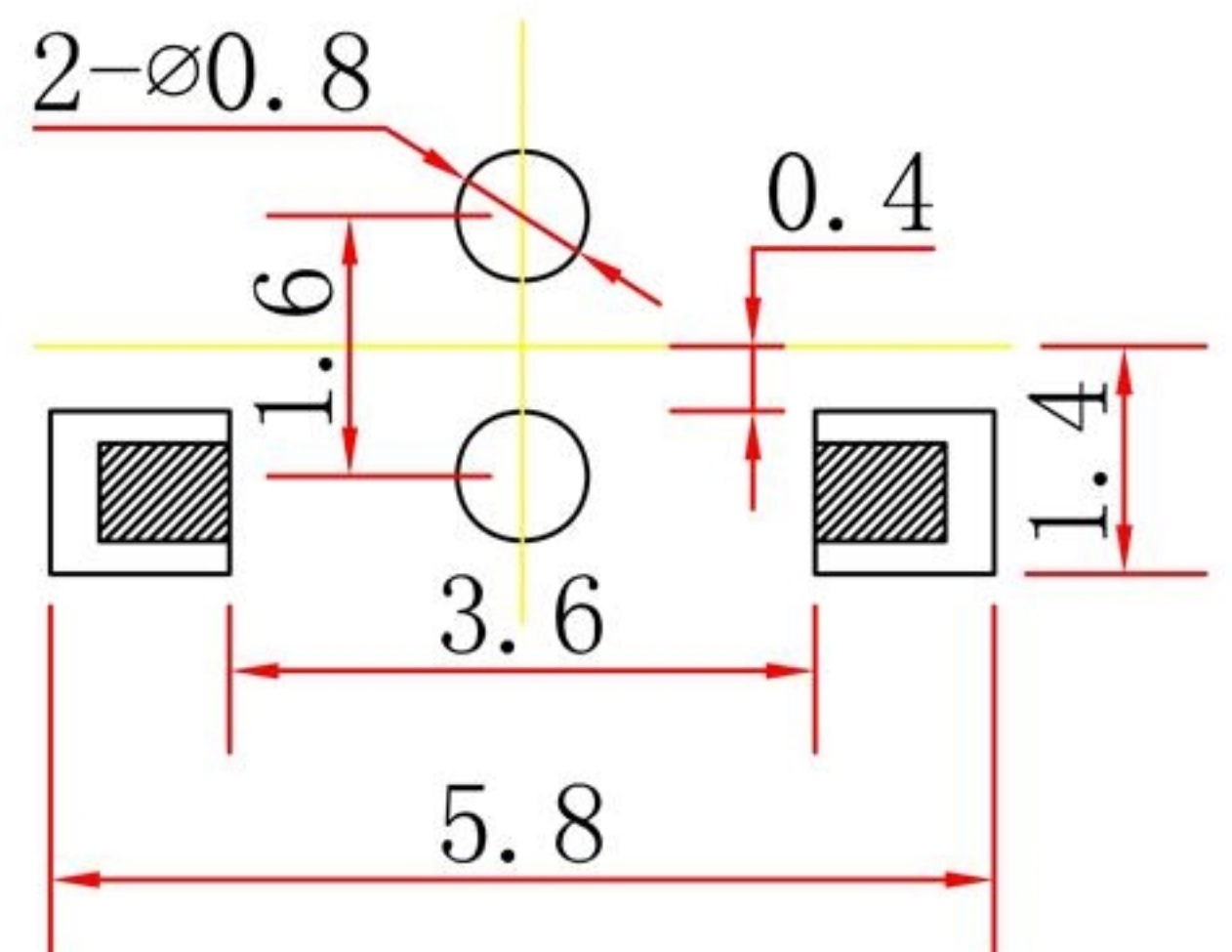
PCB板位置尺寸
