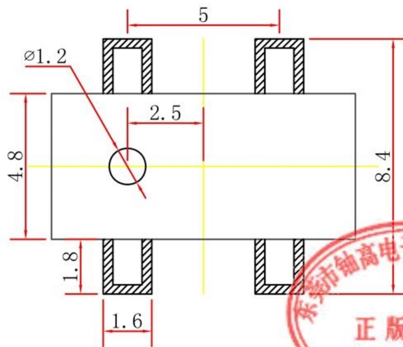
PCB板位置尺寸
