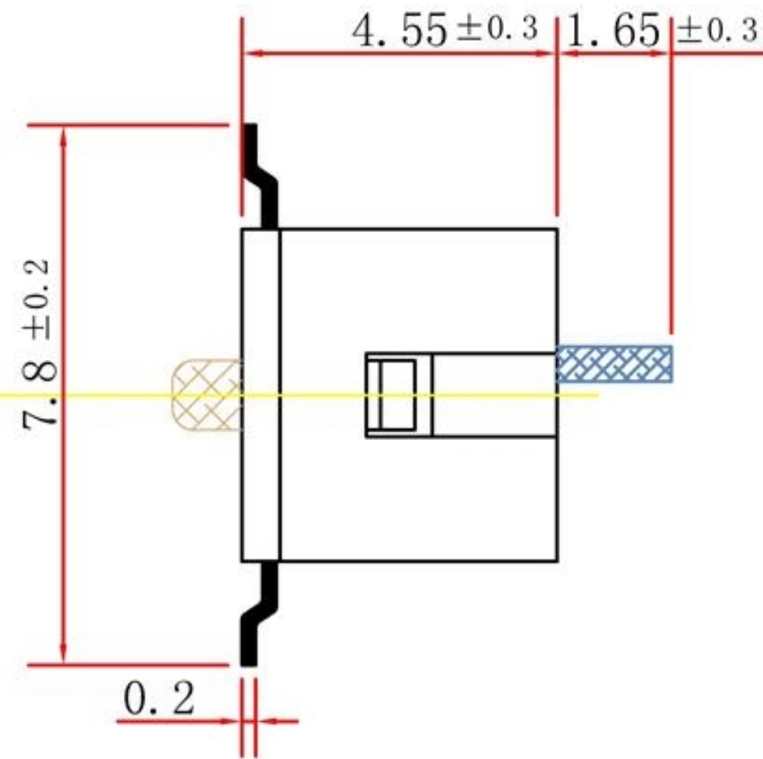
PCB板位置尺寸
