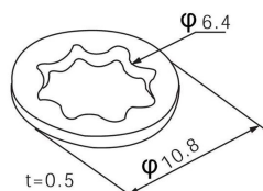
齿形华司 Zigzag Washer
