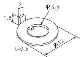
固定华司 Fix Washer
